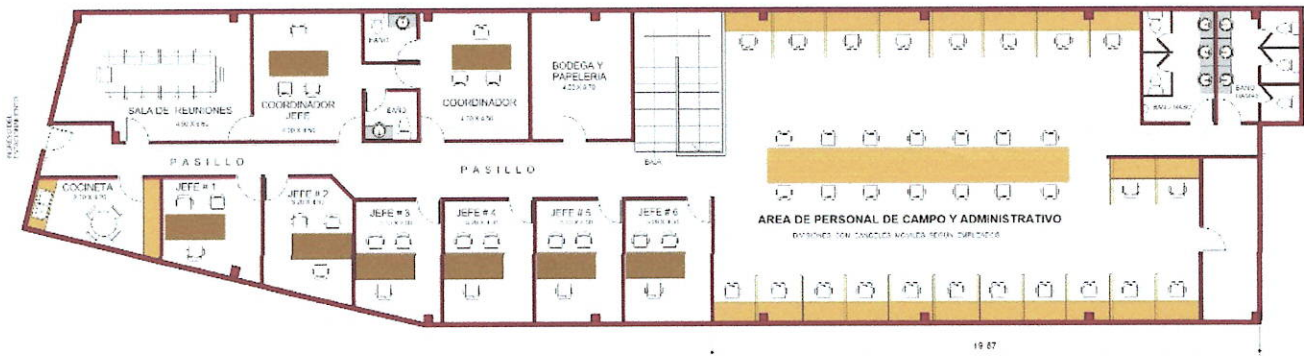
PLANTA DISTRIBUTIVA SEGUNDO PISO EDIFICIO PARA OFICINAS PROGRAMA REDUCCION DE PERDIDAS ENEE FRENTE A GASOLINERA UNO, JUTICALPA, OLANCHO. PROPIETARIA. AMINDA GOMEZ Y FAM.
